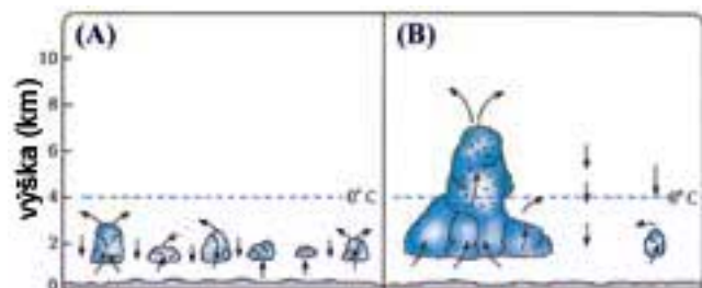
Obr. 1.19: (A) Izolované malé mraky (kupovité mraky). (B) Malé mraky stoupají směrem nahoru, až vytvoří velké mračno. Tečky naznačují kapky deště. ( The Atmosphere , Anthes a kol. str. 269).
