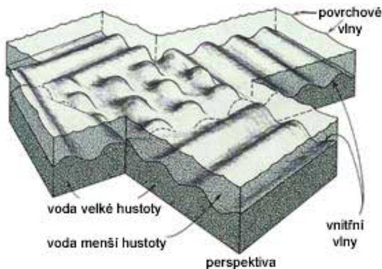
Obr. 1.16: Vnitřní vlny mezi dvěma vrstvami vody s rozdílnou hustotou. Spodní vrstva je hustší než horní. ( Oceanography , Gross, str. 204)
