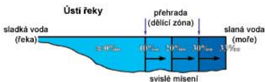
Obr. 1.14: Podélný řez ústím řeky s vyznačenými hodnotami slanosti (v promile) ilustruje přechod mezi sladkou a slanou vodou (dělicí zóna). (Upravené podle Introductory Oceanography , Thurman, str. 301)
