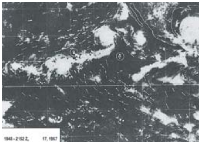
Obr. 1.17: Satelitní fotografie ukazuje mraky pohybující se směrem k místům hromadění B, C a D. Šipky označují směr větru. ( The Use of Satellite Pictures in Weather Analysis and Forecasting , Anderson a kol., str. 188)
