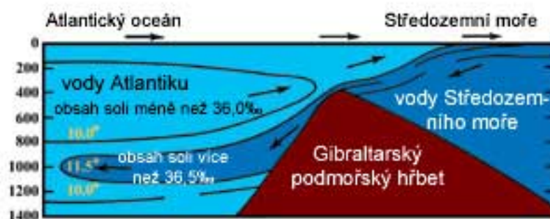
Obr. 1.13: Voda Středozemního moře, pronikající přes Gibraltarský podmořský hřbet do Atlantiku, je teplejší, řidší a má vyšší obsah solí díky bariéře, která obě moře rozděljuje. Uvedené teploty jsou ve stupních Celsia. (Upravené podle Marine Geology , Kuenen, str. 43)
