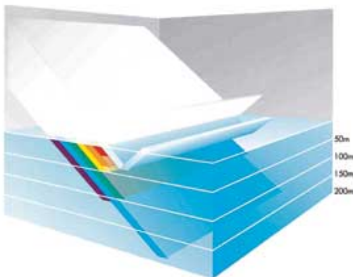
Obr. 1.15: 3 až 30% slunečního světla se odráží od hladiny moře. Potom jsou téměř všechny ze sedmi barev spektra absorbovány jedna po druhé v prvních 200 m, s výjimkou modrého světla. ( Oceans , Elder a Pernetta, str. 27)
