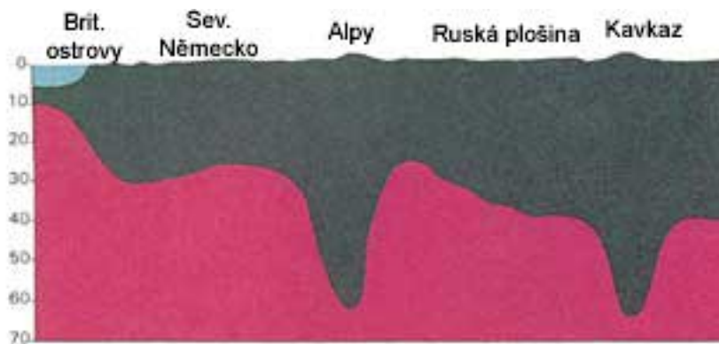
Obr. 1.8: Schematický řez. Hory jako kůly mají hluboké kořeny zakotvené v zemi. ( Anatomy of the Earth , Cailleux, str. 220)
